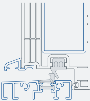
Variante ouvrant vers l'intérieur
